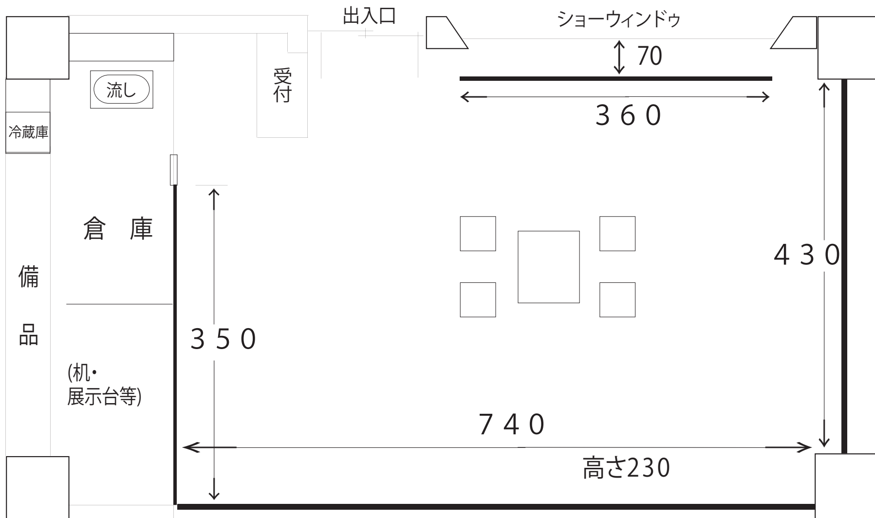
■市立ギャラリーいけだ展示室内平面図(45平方メートル)
